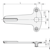
Optional cam S3C8800
