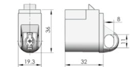
Optional profile insert TC06-1
